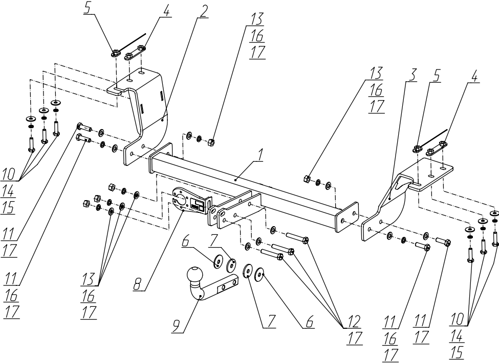
Схема монтажа
